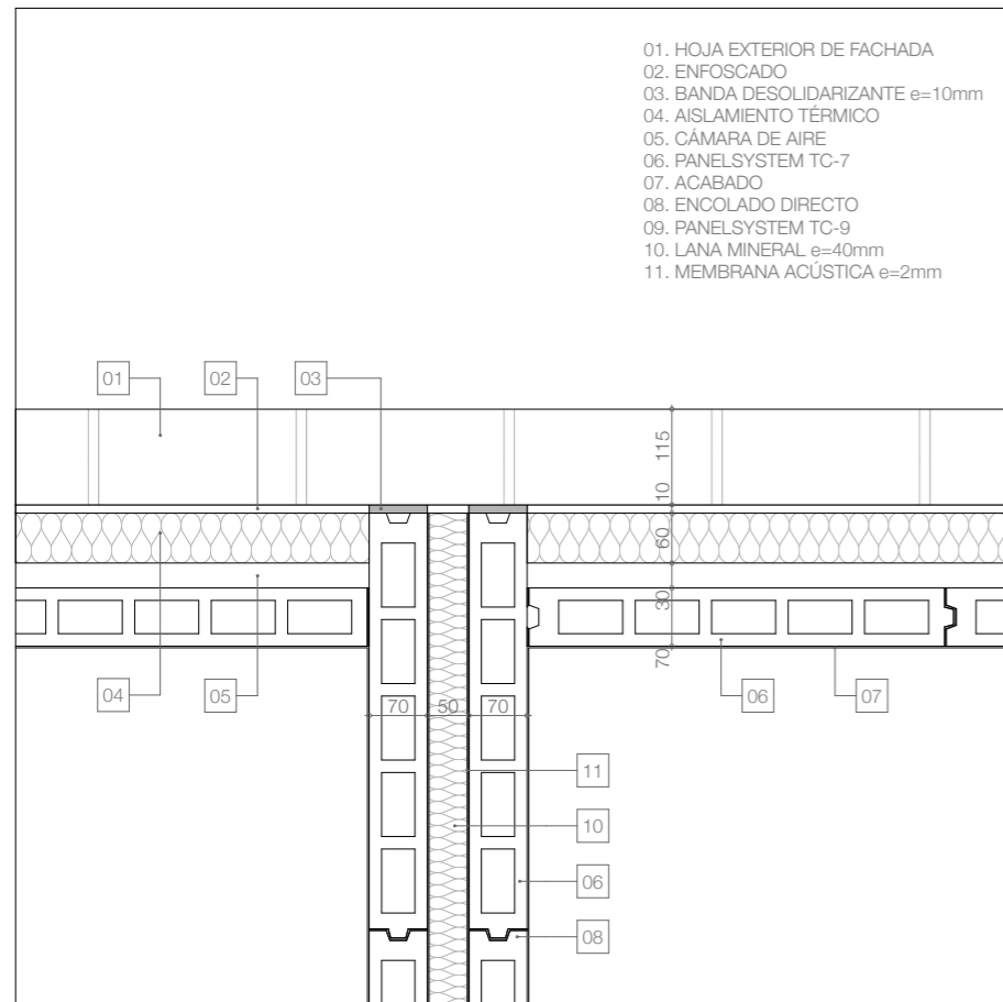
ENCUENTRO DE PARTICION INTERIOR CON FACHADA. TC7+TC7
