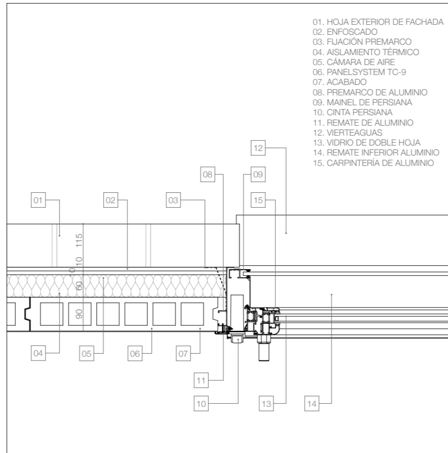
SECCIÓN HORIZONTAL POR JAMBA DE CARPINTERÍA DE ALUMINIO. TRASDOSADO TC9
