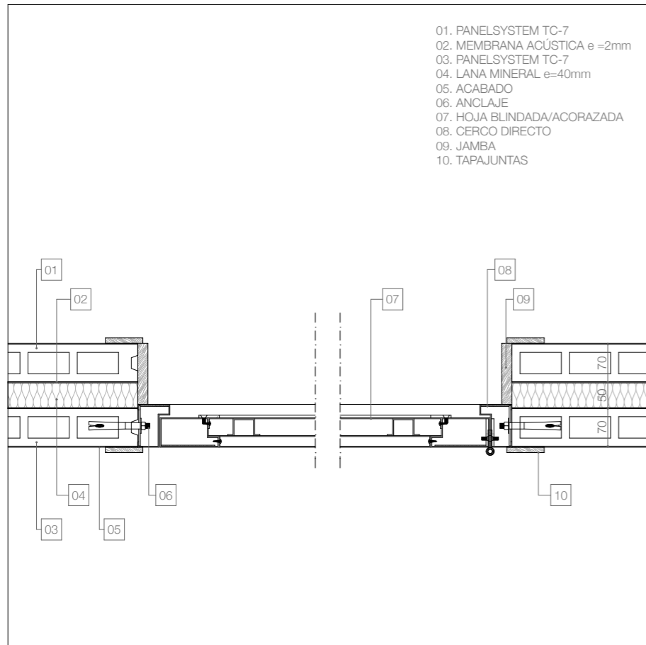
SECCIÓN HORIZONTAL. MEDIANERÍA TC-7+TC-7 CON PUERTA DE ENTRADA
