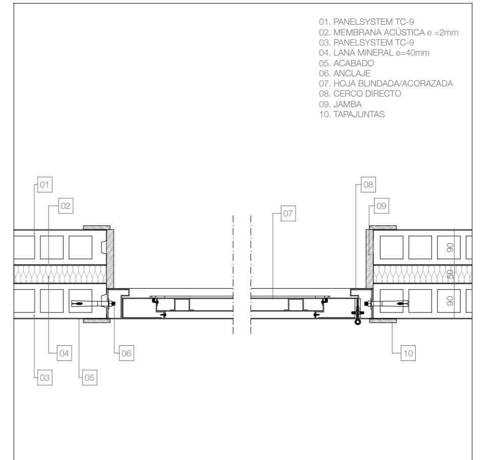
SECCIÓN HORIZONTAL. MEDIANERÍA TC-9+TC-9 CON PUERTA DE ENTRADA
