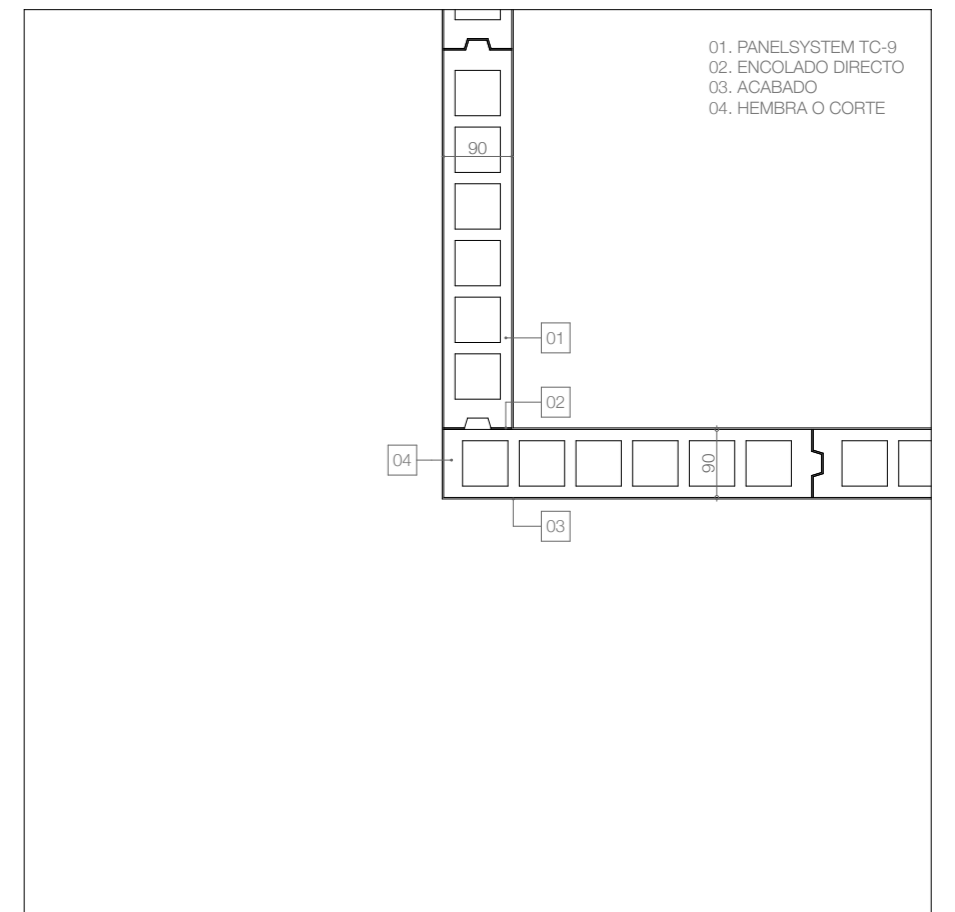
ENCUENTRO DE PARTICION INTERIOR EN ESQUINA. TC9
