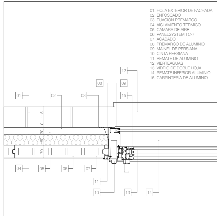
SECCIÓN HORIZONTAL POR JAMBA DE CARPINTERÍA DE ALUMINIO. TRASDOSADO TC7
