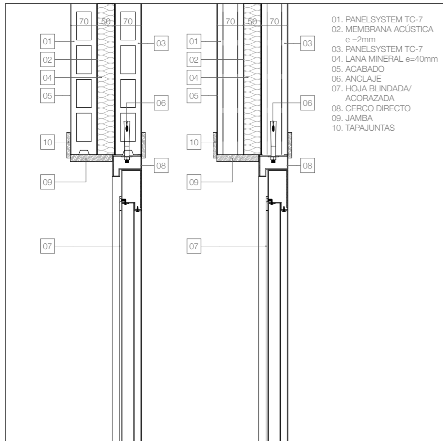
SECCIÓN VERTICAL. MEDIANERÍA TC-7+TC-7 CON PUERTA DE ENTRADA
