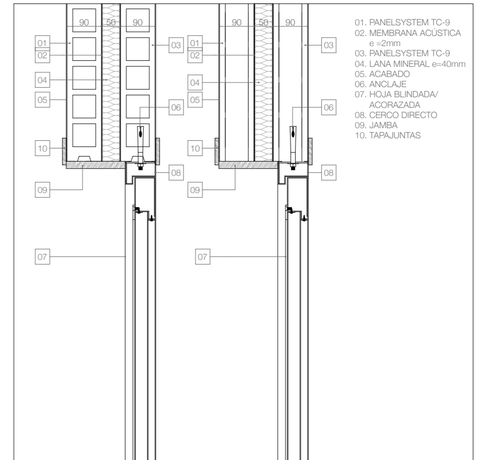
SECCIÓN VERTICAL. MEDIANERÍA TC-9+TC-9 CON PUERTA DE ENTRADA
