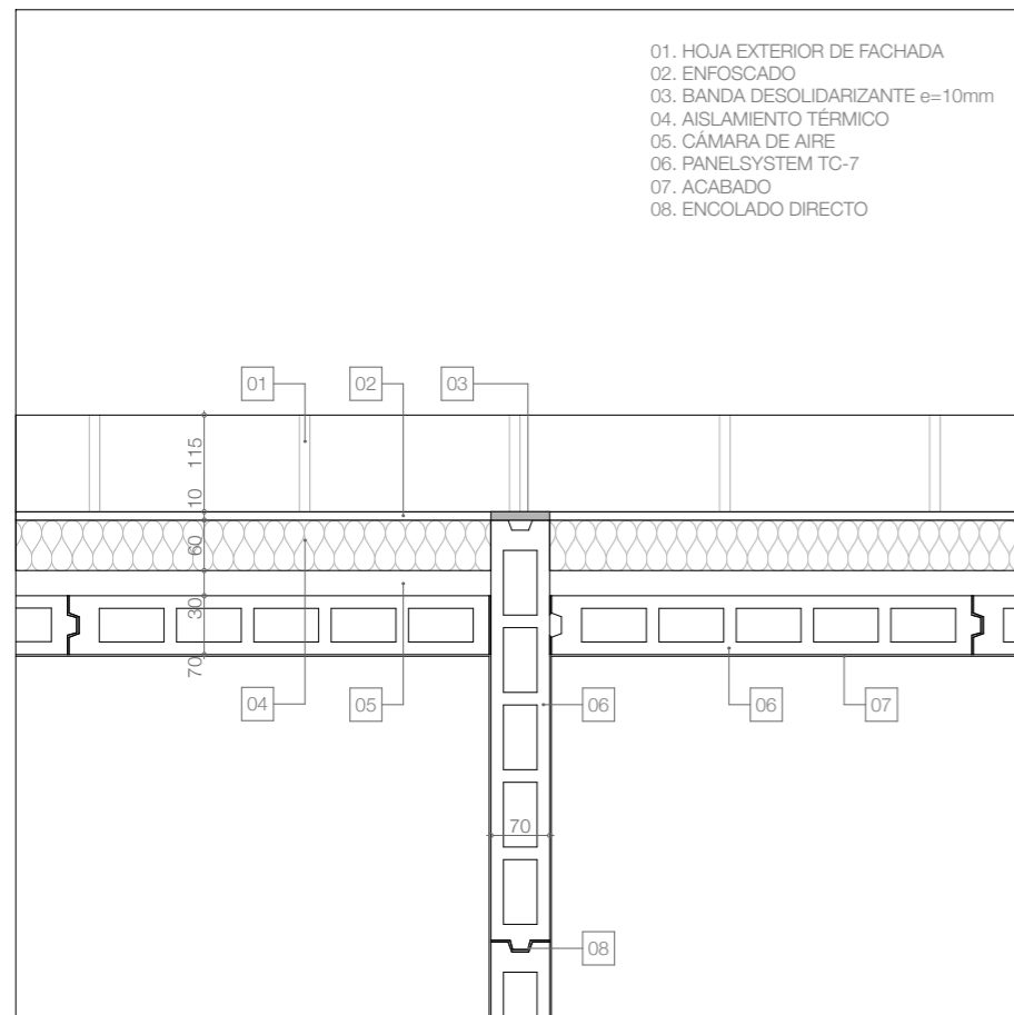
ENCUENTRO DE PARTICION INTERIOR CON HOJA EXTERIOR DE FACHADA. TC7
