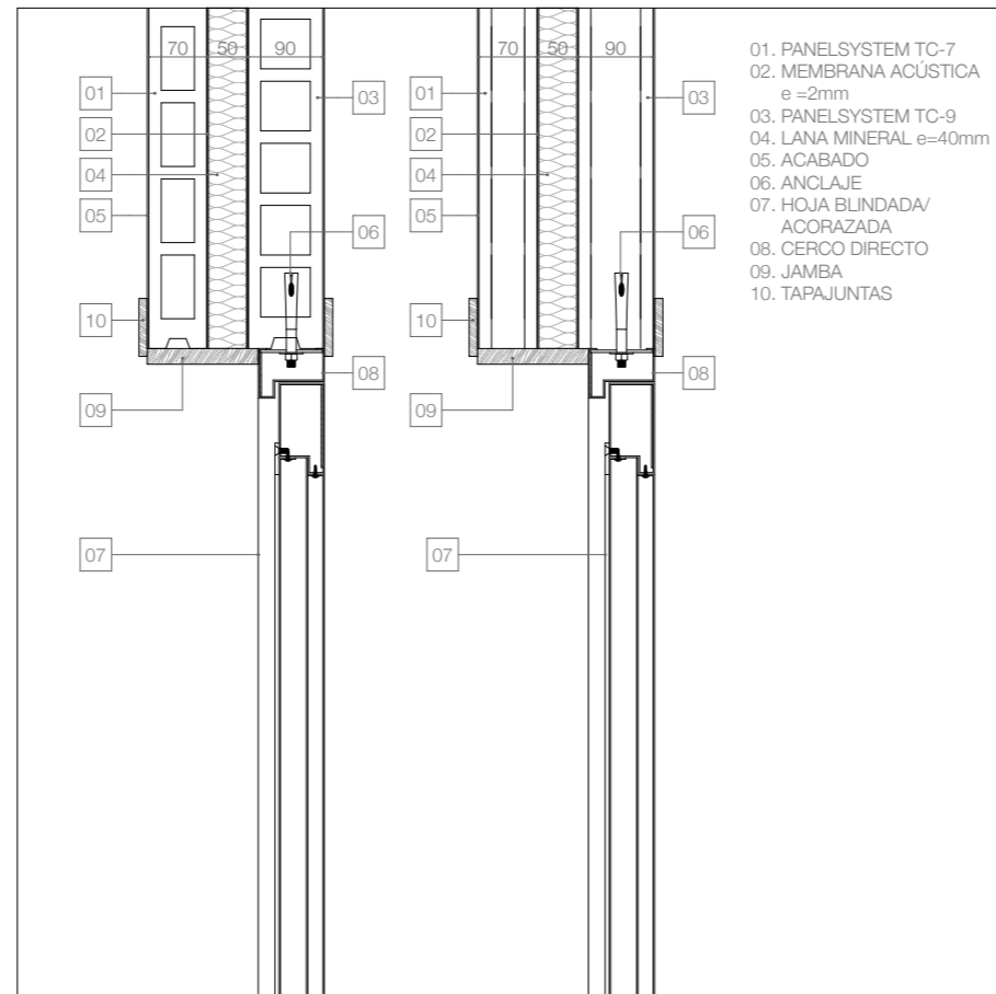
SECCIÓN VERTICAL. MEDIANERÍA TC-7+TC-9 CON PUERTA DE ENTRADA
