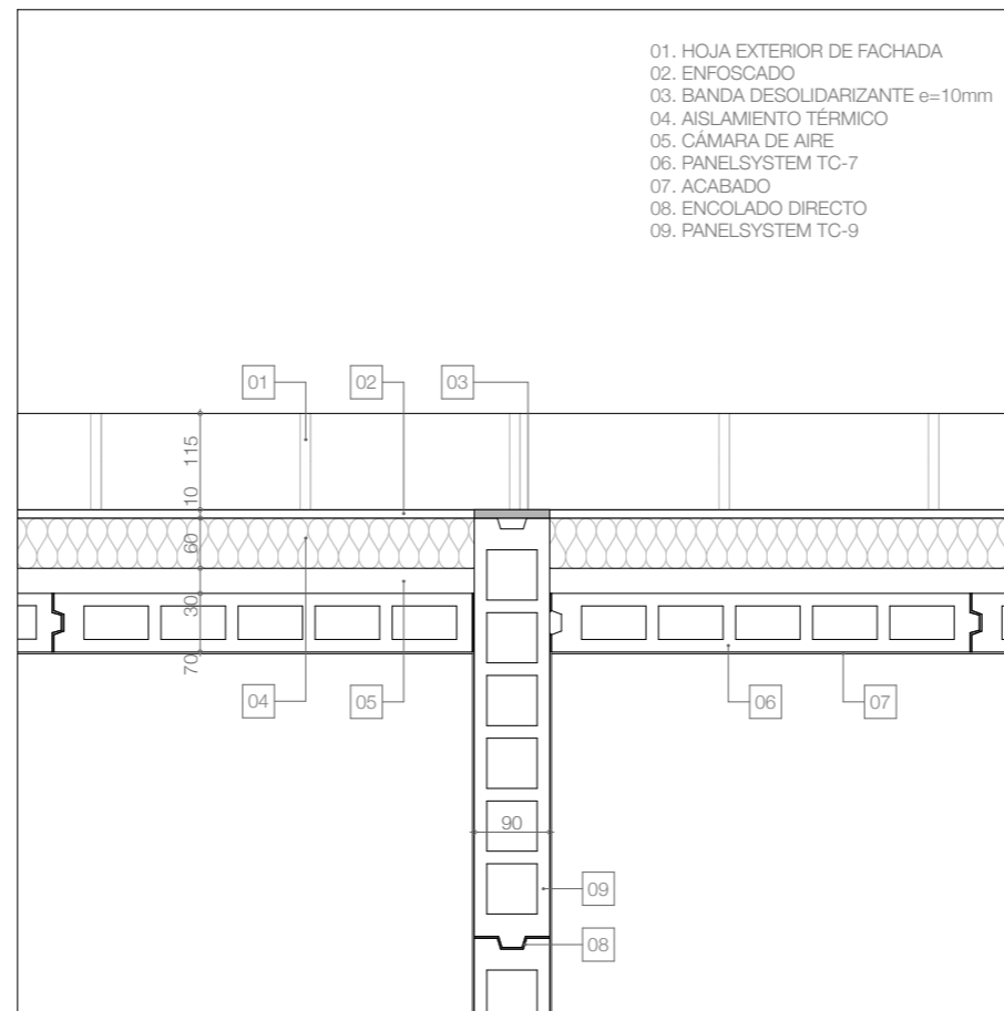
ENCUENTRO DE PARTICION INTERIOR CON HOJA EXTERIOR DE FACHADA. TC9
