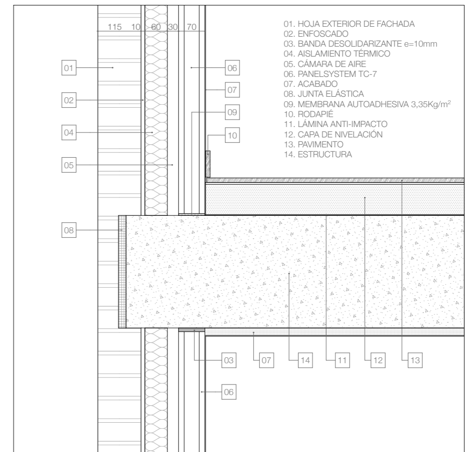
SECCIÓN VERTICAL POR ARRANQUE Y REMATE DE PANELES DE TRASDOSADO
