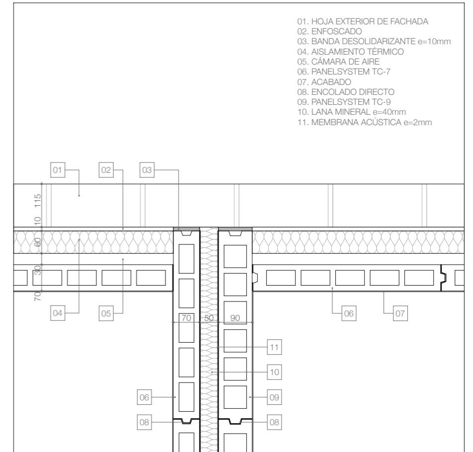
ENCUENTRO DE PARTICION INTERIOR CON FACHADA. TC7+TC9
