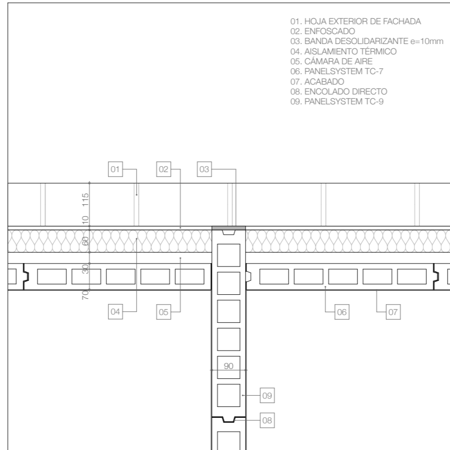
ENCUENTRO DE PARTICION INTERIOR CON FACHADA. TC9
