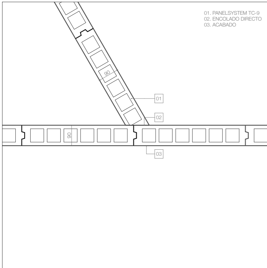
ENCUENTRO DE PARTICION INTERIOR EN ANGULO. TC9
