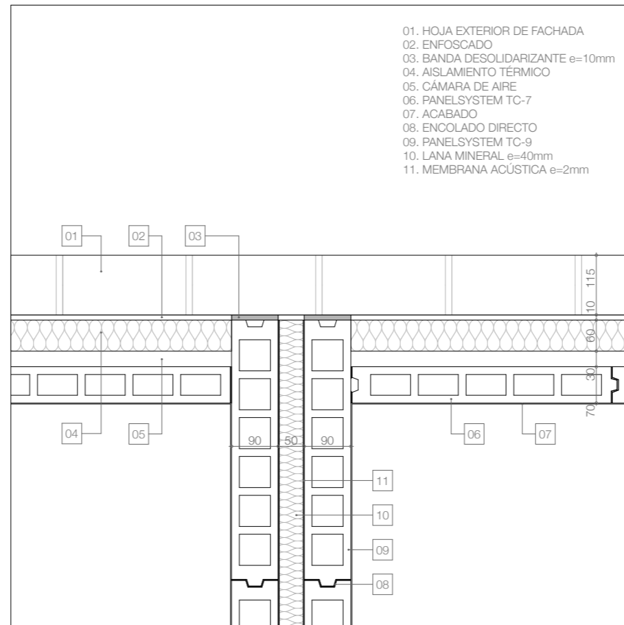
ENCUENTRO DE PARTICION INTERIOR CON FACHADA. TC9+TC9
