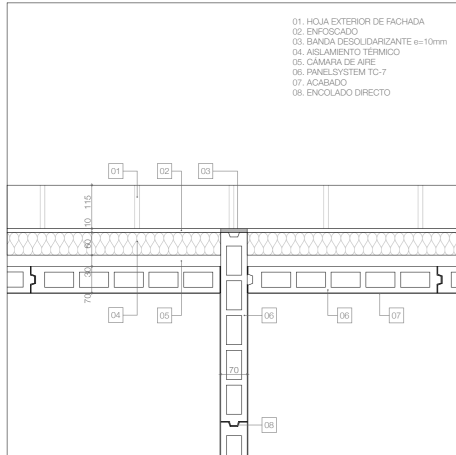
ENCUENTRO DE PARTICION INTERIOR CON FACHADA. TC7
