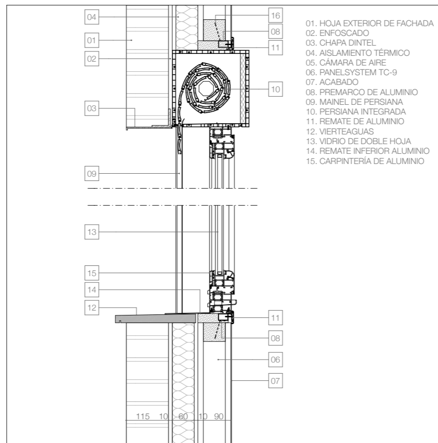
SECCIÓN VERTICAL POR VENTANA DE CARPINTERÍA DE ALUMINIO. TRASDOSADO TC9
