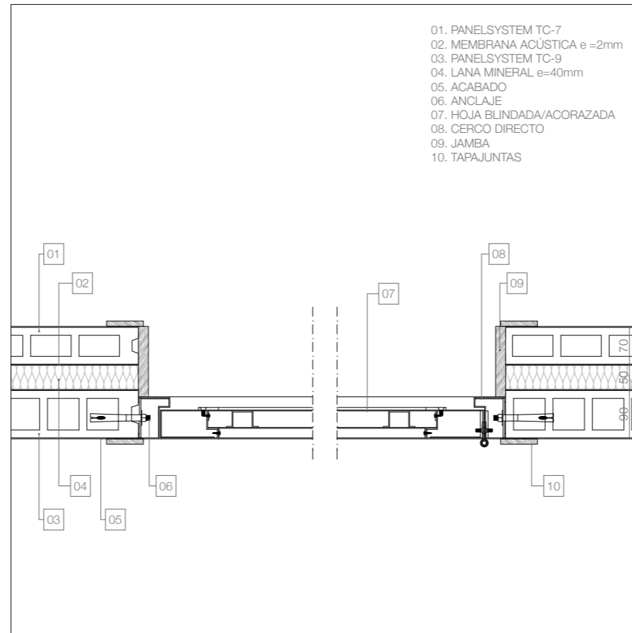
SECCIÓN HORIZONTAL. MEDIANERÍA TC-7+TC-9 CON PUERTA DE ENTRADA
