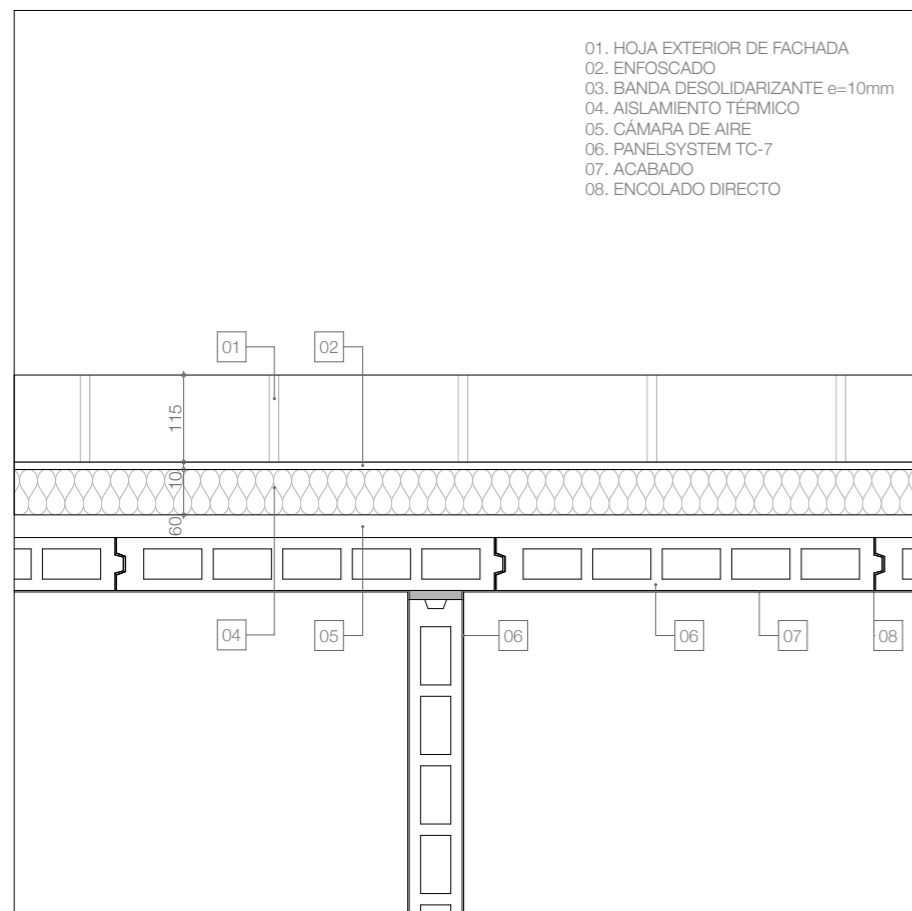
ENCUENTRO DE PARTICION INTERIOR CON TRASDOSADO. TC7
