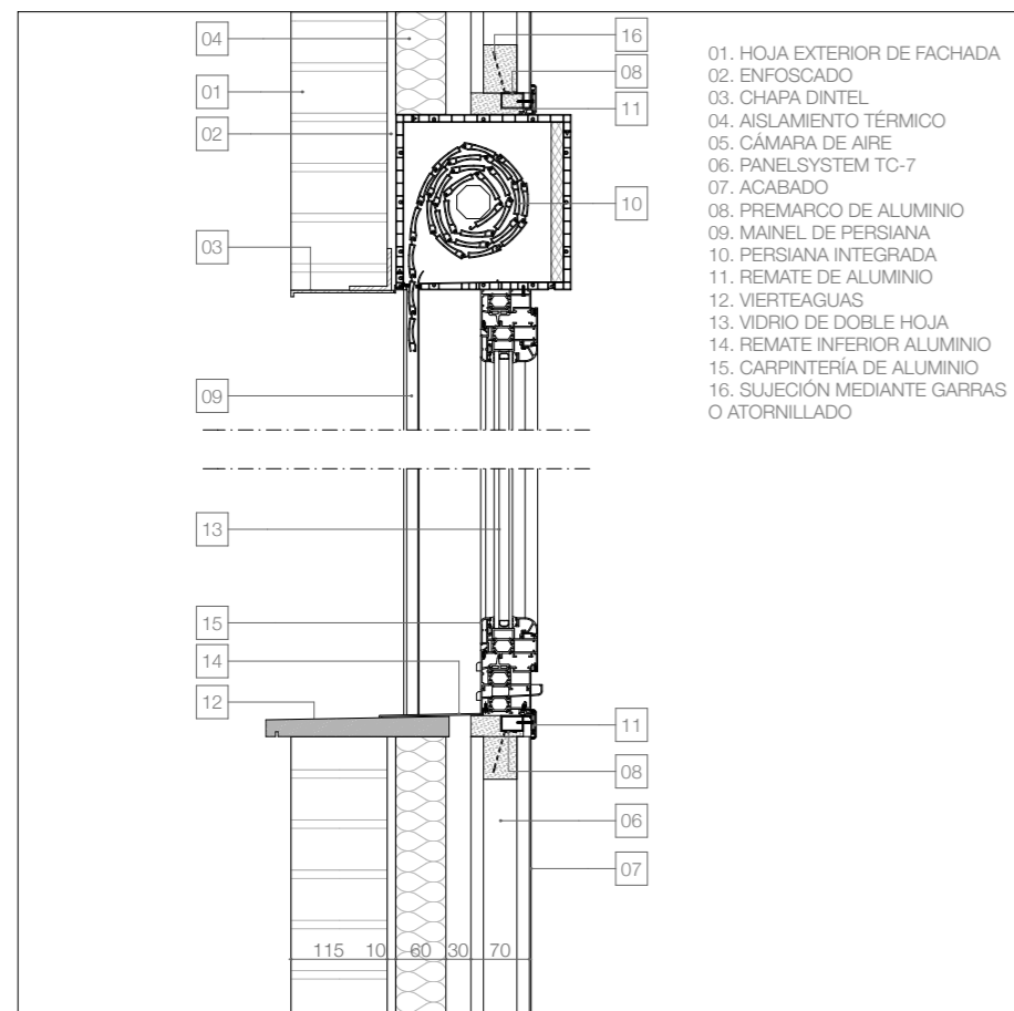
SECCIÓN VERTICAL POR VENTANA DE CARPINTERÍA DE ALUMINIO. TRASDOSADO TC7
