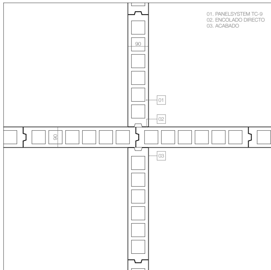
ENCUENTRO DE PARTICION INTERIOR EN CRUZ. TC9
