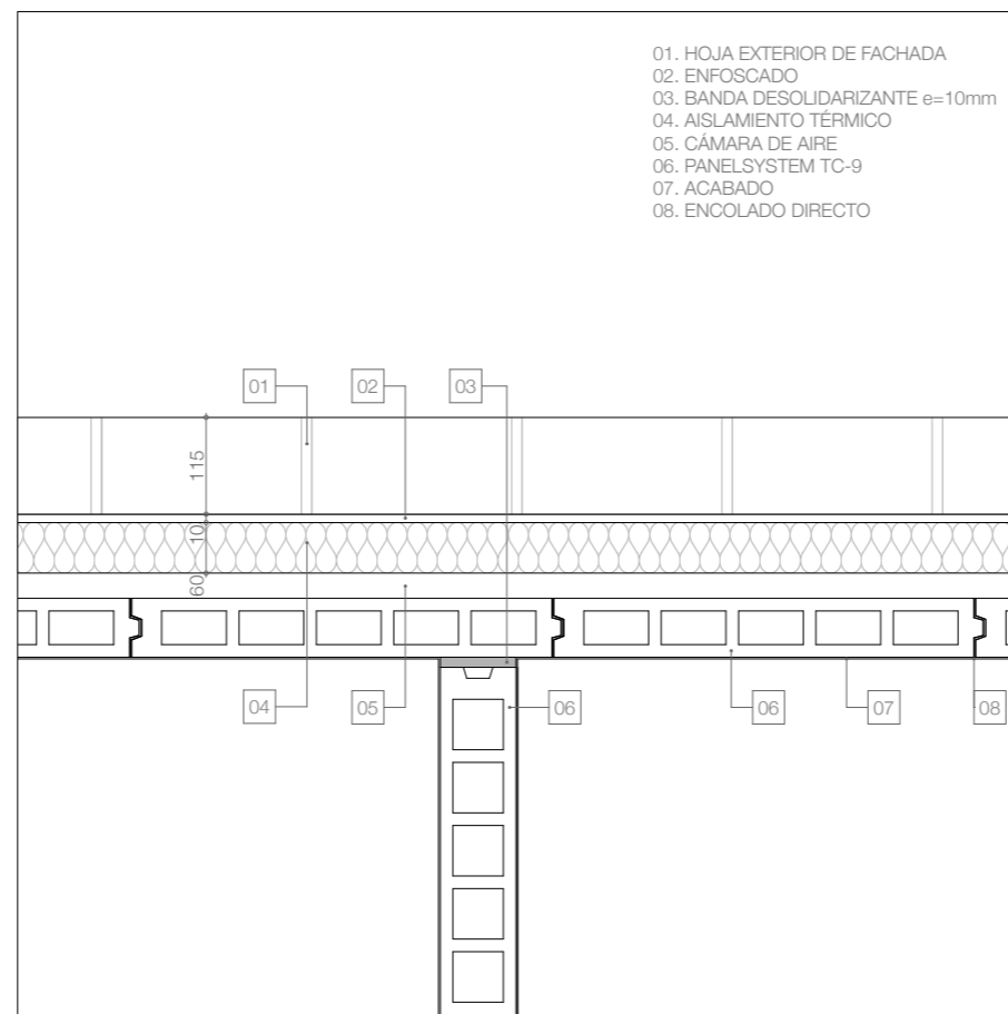
ENCUENTRO DE PARTICION INTERIOR CON TRASDOSADO. TC9
